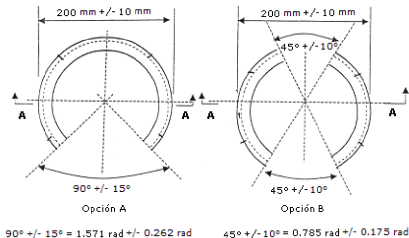
Figura 7 - Alternativas de cuello protector para recipiente portátil
