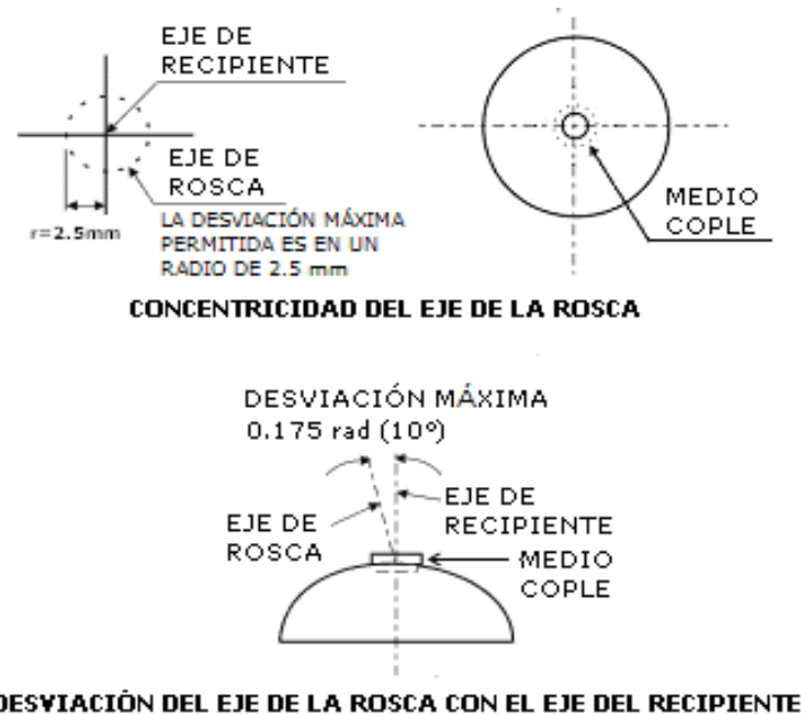
Figura 13 - Concentricidad y desviación del medio cople con el recipiente
