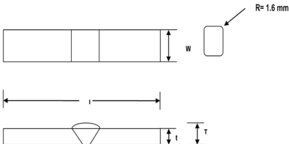
Figura 17 - Probeta de doblez guiado
