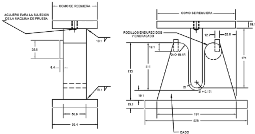
Figura 18 - Dispositivo estandarizado para doblez guiado
